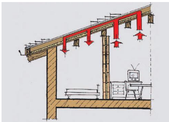
• Trasmissione laterale del rumore attraverso l'intercapedine di ventilazione (a sinistra); taglio acustico con materiale fibroso in corrispondenza delle partizioni verticali (a destra).
