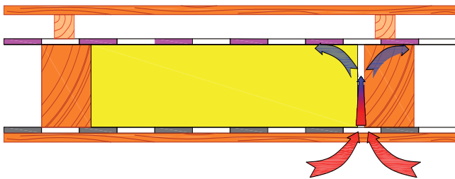
• Convezione el vapore attraverso giunti aperti.
