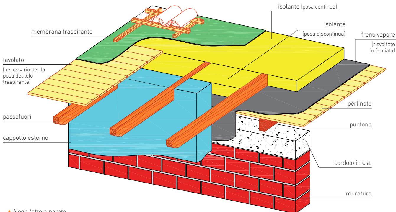
• Nodo tetto a parete.
