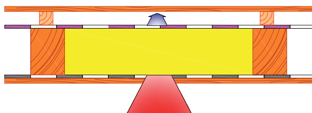
• Diffusione del vapore attraverso gli strati della copertura.
