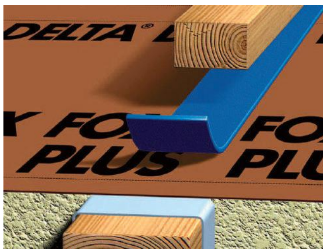
• Posa della guarnizione punto chiodo (foto sopra e sotto).
