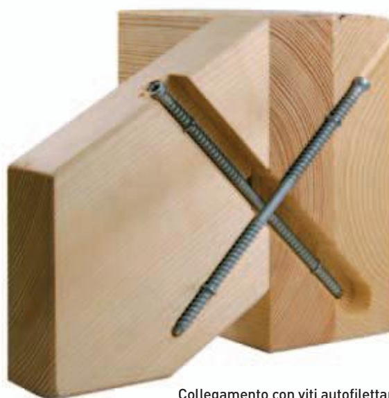
Collegamento con viti autofilettanti
