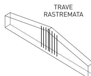
• Esempi di rinforzo strutturale mediante applicazione di viti a tutto filetto per scongiurare la rottura per trazione ortogonale.
