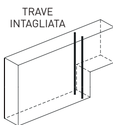
• Esempi di rinforzo strutturale mediante applicazione di viti a tutto filetto per scongiurare la rottura per trazione ortogonale.
