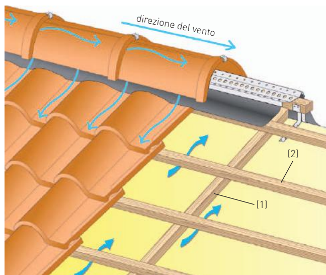
• Doppia listellatura per macroventilazione.
