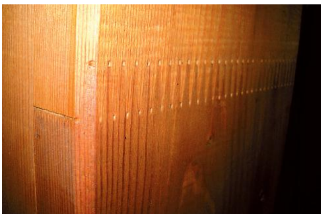
• Particolare giunto a pettine.
