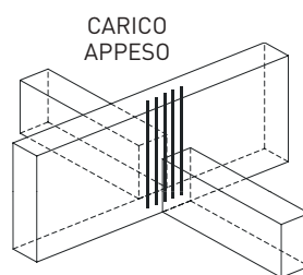
• Esempi di rinforzo strutturale mediante applicazione di viti a tutto filetto per scongiurare la rottura per trazione ortogonale.
